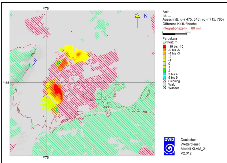
Abbildung 34: Differenz Kaltfluthöhe zwischen Soll- und Istzustand nach 60 Minuten
