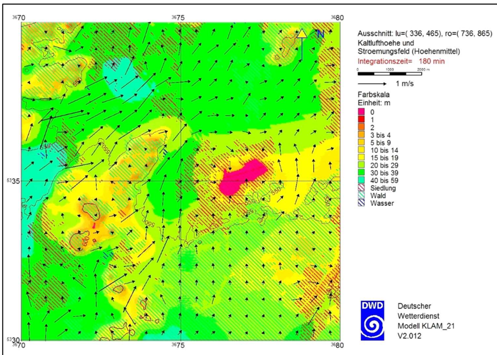
Abbildung 26: Kaltluflthöhe/Strömungsfeld 180 Minuten (3 Stunden) nach Simulationsstart
