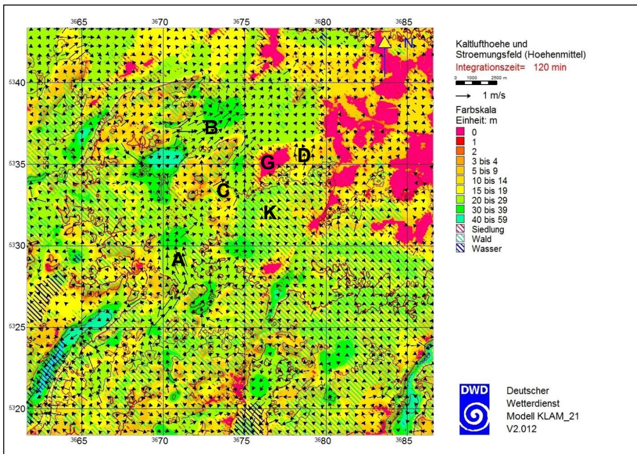
Abbildung 23: Kaltluflhöhe/Strömungsfeld 120 Minuten (2 Stunden) nach Simulationsstart (komplettes Rechengebiet)
