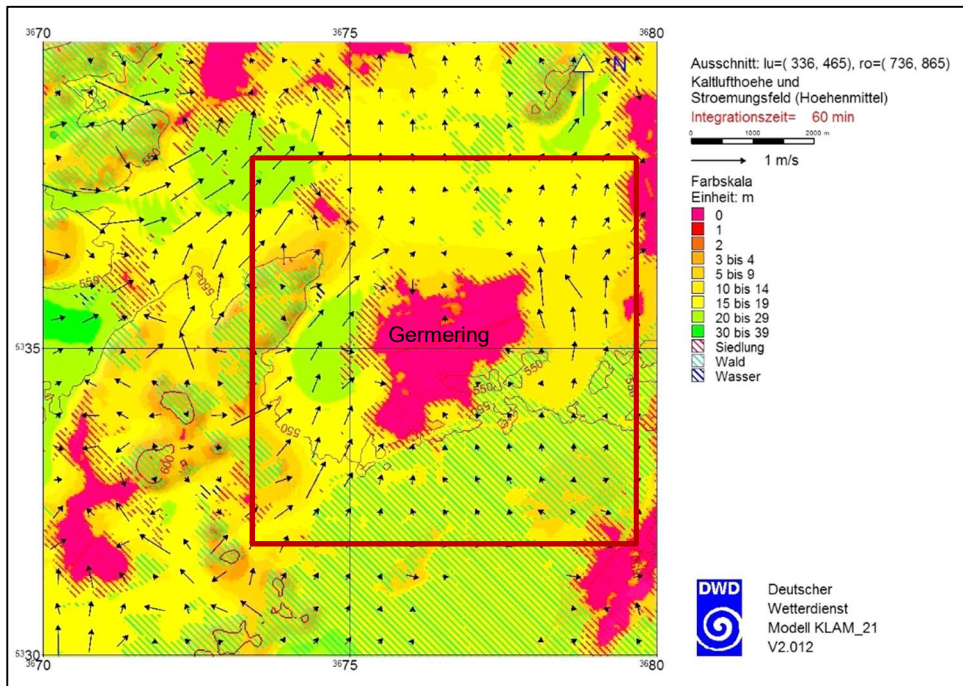
Abbildung 24: Kaltluflhöhe/Strömungsfeld 60 Minuten nach Simulationsstart für Ausschnitt A sowie Lage Ausschnitt B (roter Rahmen)
