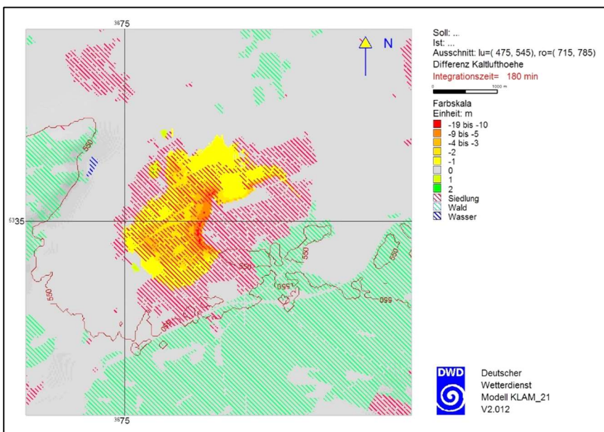
Abbildung 35: Differenz Kaltfluthöhe Soll- minus Istzustand 180 Minuten nach Simulationsstart
