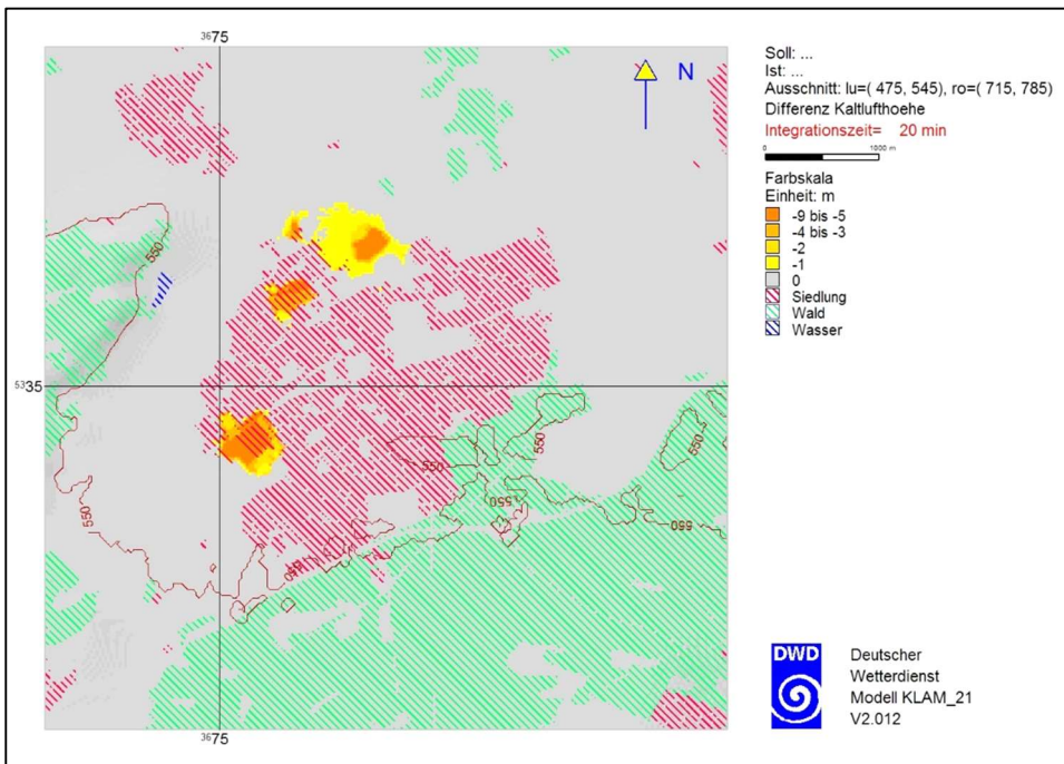
Abbildung 33: Differenz Kaltluflthöhe zwischen Soll- und Istzustand nach 20 Minuten
