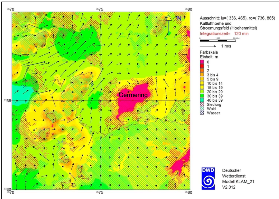
Abbildung 25: Kaltluflthöhe/Strömungsfeld 120 Minuten (2 Stunden) nach Simulationsstart
