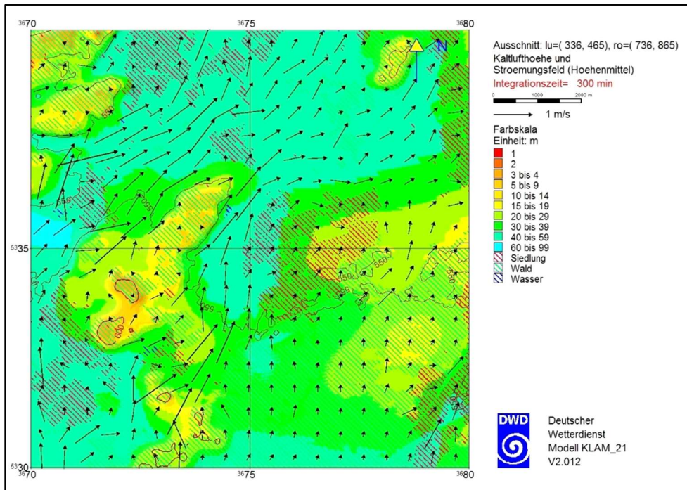
Abbildung 27: Kaltluflthöhe/Strömungsfeld 300 Minuten (5 Stunden) nach Simulationsstart
