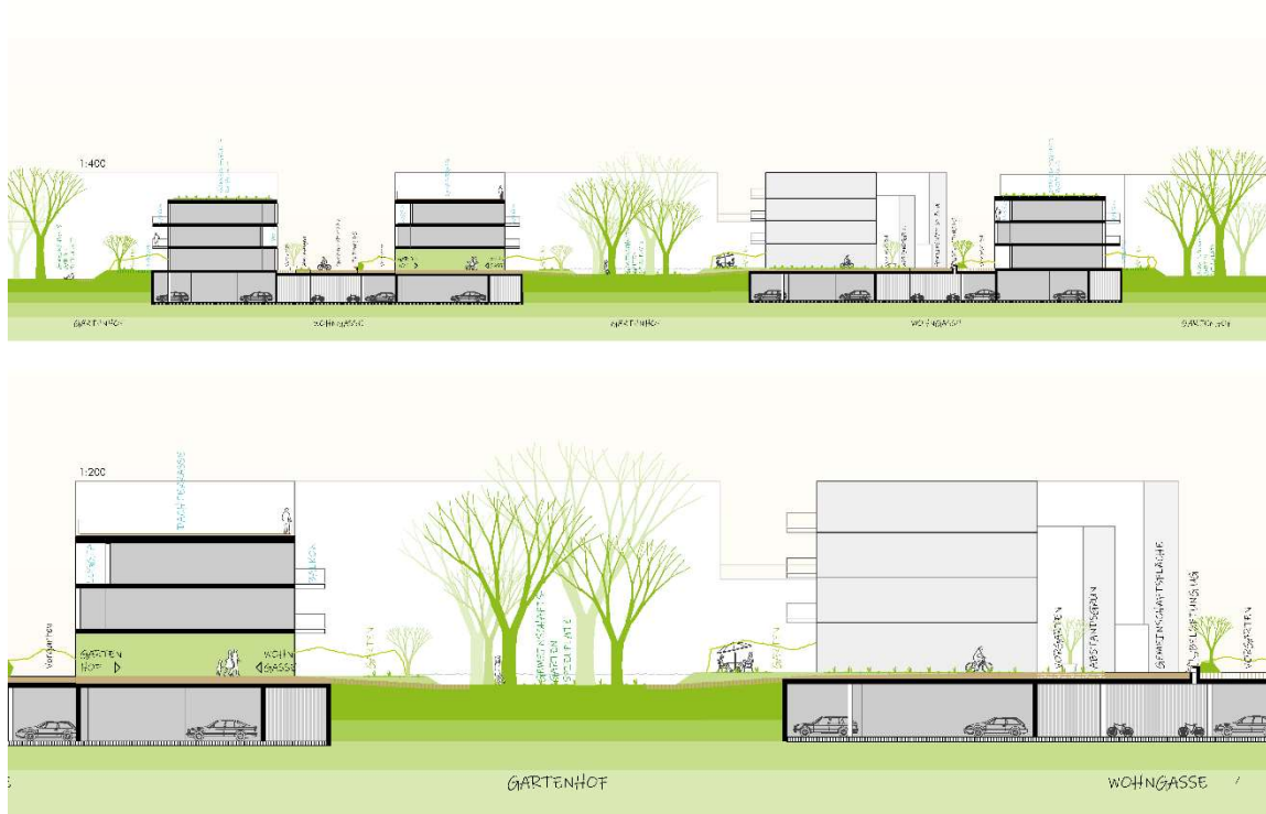
Abb. 11: Schnitt in Ost-Westrichtung (ohne Maßstab)
