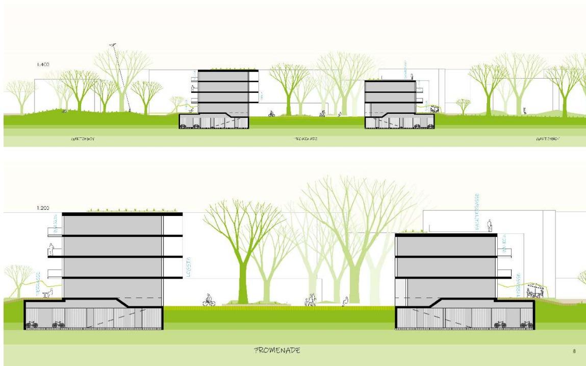
Abb. 12: Schnitt in Nord-Südrichtung (ohne Maßstab)
